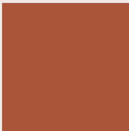
Danthron BP
