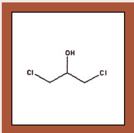
1,3-Dichloroisopropanol
